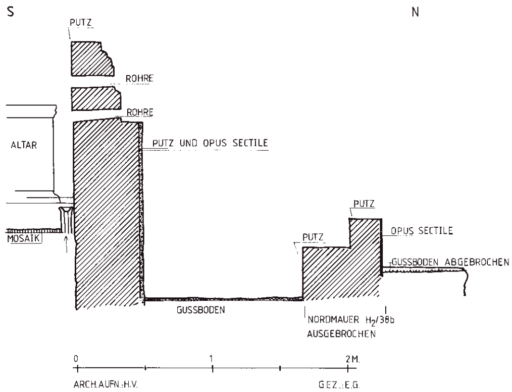
Abb. 139: 38e, Badebecken, N-S-Schnitt
